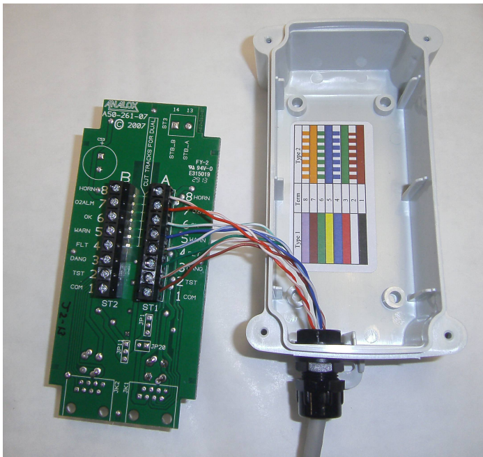
Fernalarmgeber Klemme Analox 50 / 50M
